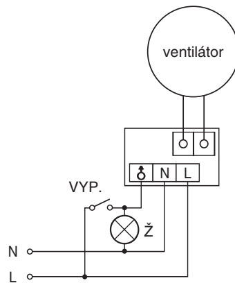
Zapojení s hygrostatem
