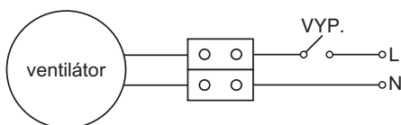
Standardní zapojení
