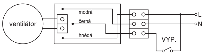
Zapojení s časovým spínačem na vypínač
