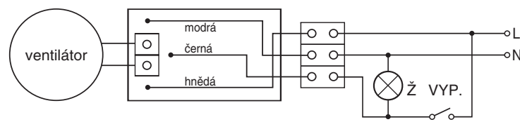
Zapojení s časovým spínačem na světelný okruh
