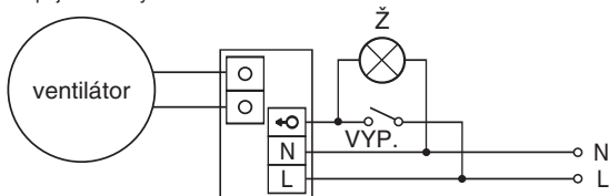
Zapojení dvourychlostních ventilátorů
