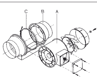
A – vyjímatelná ventilátorová jednotka s motorem, oběžným kolem a svorkovnicí B – montážní konzola s přípojevacími hrdly C – ocelová spona pro spojení jednotky s montážní konzolou
