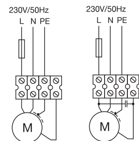
schéma elektrického zapojení
