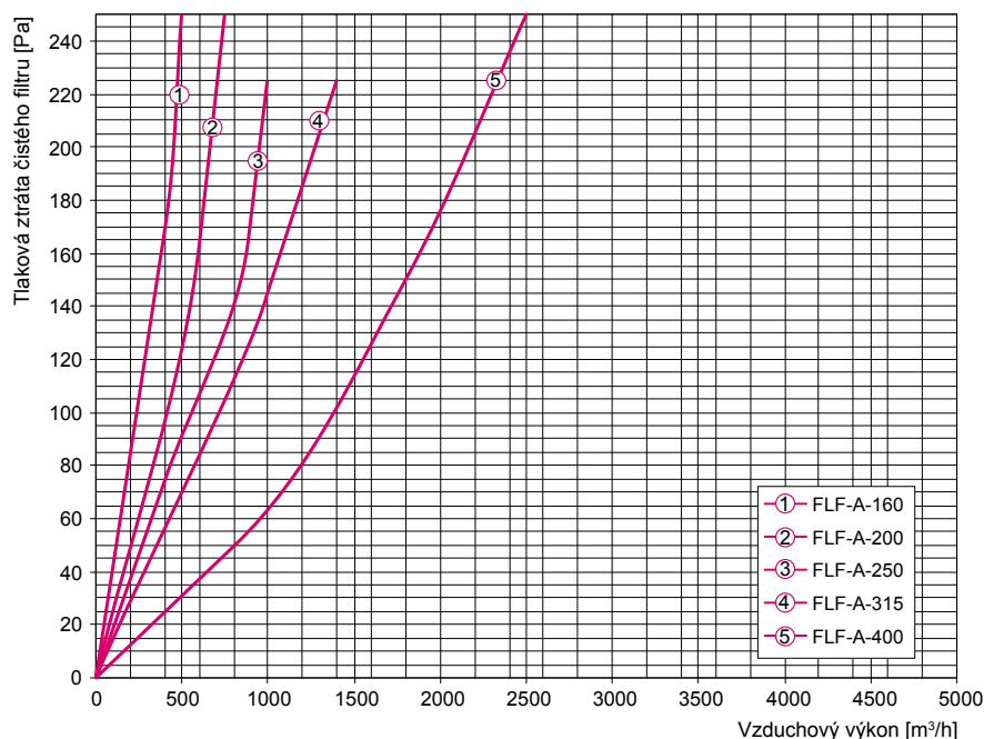
Graf tlakové ztráty filtračního boxu FLF-A třída filtrace F
