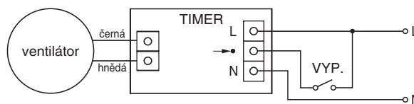
Zapojení s časovým spínačem
