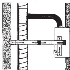
Montáž do byt. jádra - provedení UP
